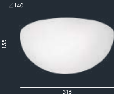
A.7235 E27 1x75W max ⊕ ∇ IP20 CE
